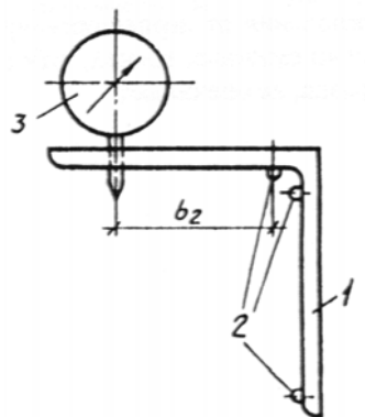
1 - корпус (угольник) ; 2 - опора; 3 - индикатор; b_2 - база прибора
